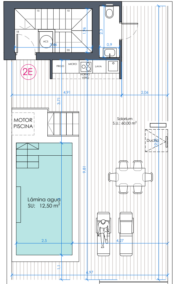
Planta Solarium
