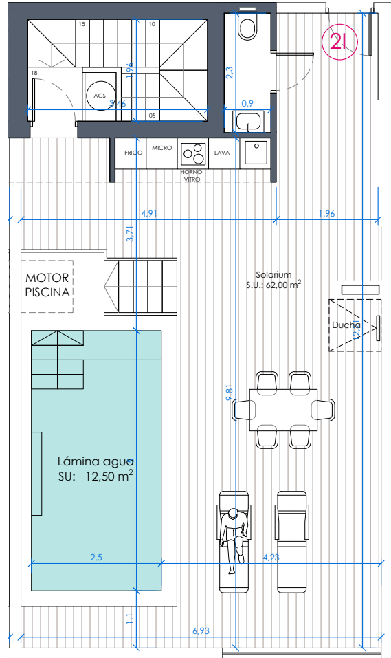
Planta Solarium
