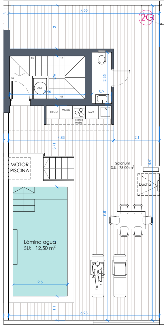
Planta Solarium
